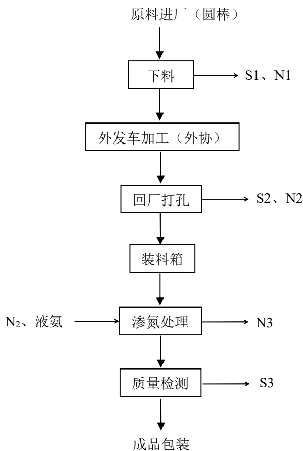
图 2-2 塔机销轴生产工艺流程图
